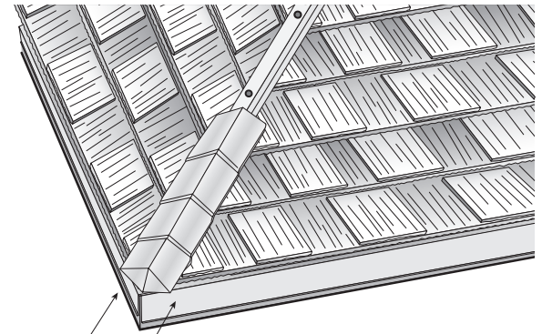
Sujetadores en ambos lados de limatesas y cumbresras
