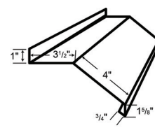
LG 147 F&J SOFFIT
