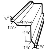
LG 125 9/16" DOOR JAMB
