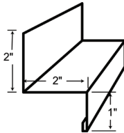
LG 130 SLIDING DOOR DRIP CAP
